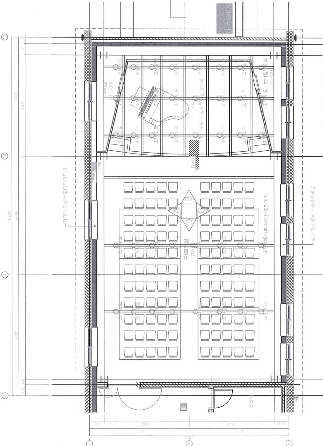
2층 다목적실 평면도 SCALE : 1/60 AREA : 139.50m 2 (42.20py)
